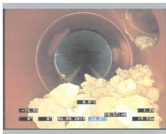
Fotografie: 16_1_2B06082019_110628_A.JPG 20,24m, Usazeniny: Tvrdý nebo zhuštěný materiál, 35% výšky potrubí, od 4 do 8 hodin, na spoji potrubí / Koniec pozorovania
