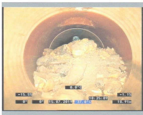
Fotografie: 1_1_1C115072019_103350_A.JPG 19,38m, Usazeniny: hrubý materiál, 80% výšky potrubí, od 2 do 11 hodin / Koniec pozorovania ,Neda sa prejsť , Makadam
